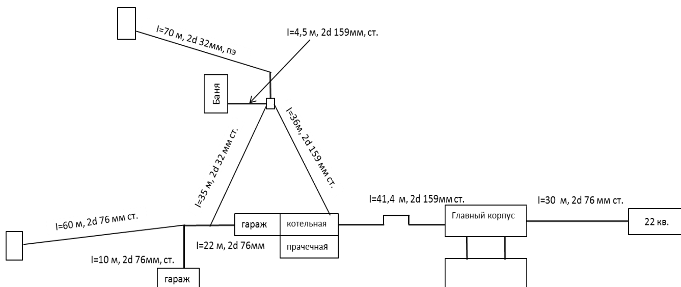
Схема 2 Тепловые сети АСУСО «Екатерининский ДИ»
